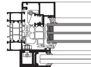
Verdeckter Flügel, Rahmfalzhöhe: 44 mm
